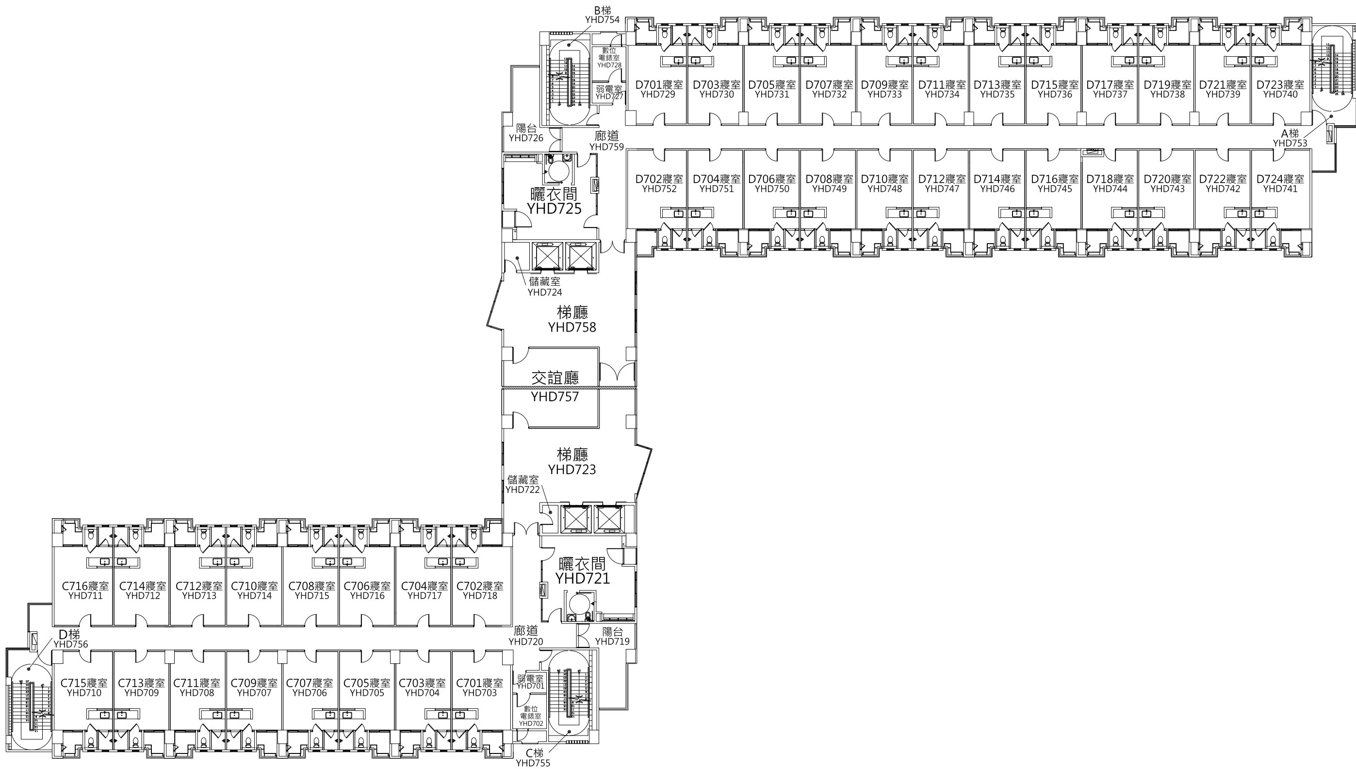
七層平面圖
