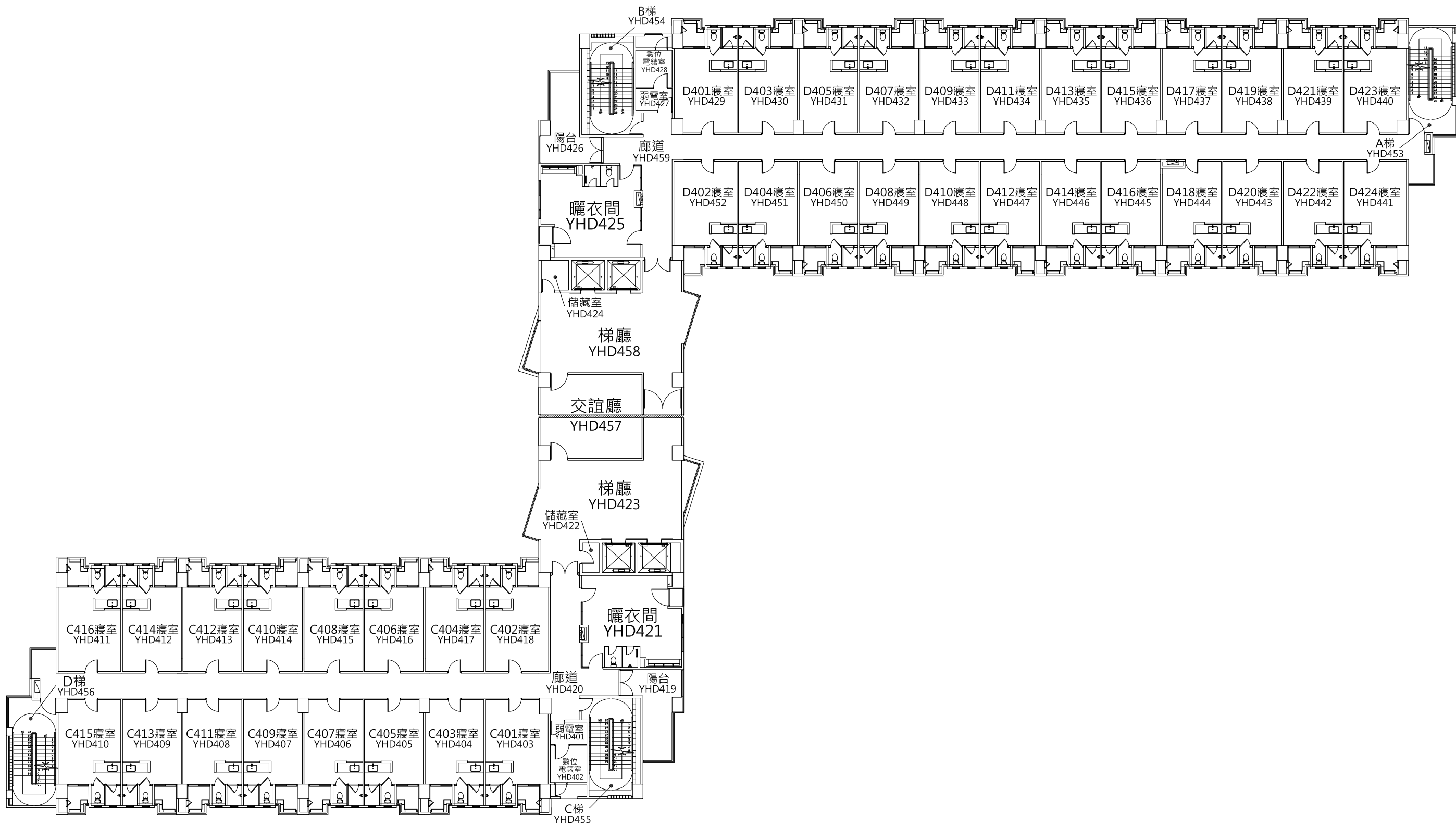
四層平面圖
